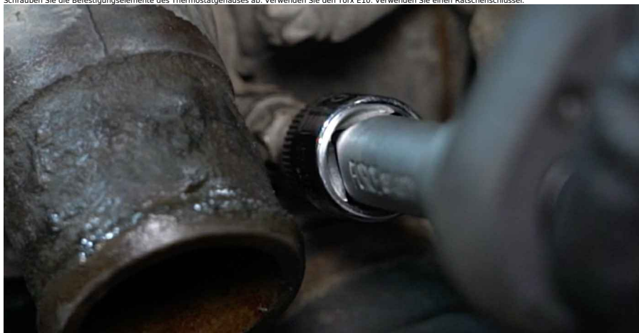
21 Entfernen Sie das Thermostatgehäuse zusammen mit dem Thermostat.
