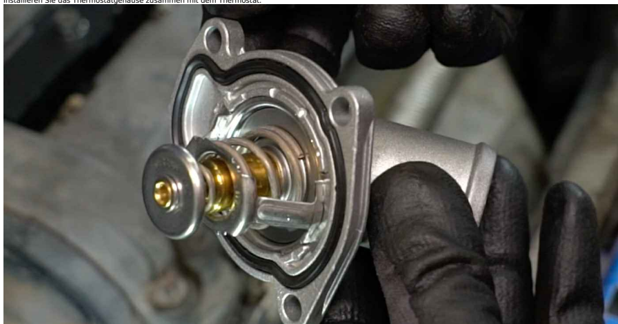
26 Bringen Sie den Gummistreifen an.
