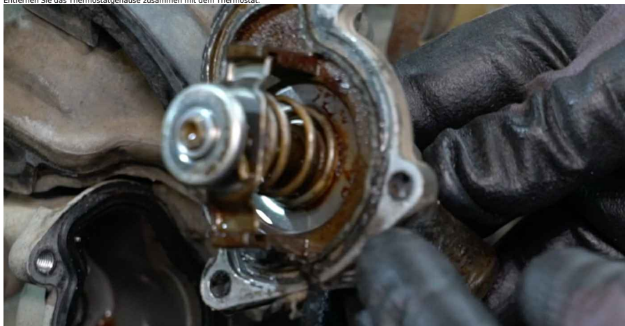
22 Decken Sie den Montagesitz des Thermostatgehäuses mit einem Mikrofasertuch ab, um zu verhindern, dass Schmutz und Fremdkörper in das System gelangen.
