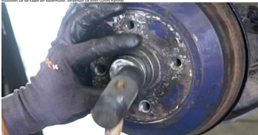
35 Behandeln Sie die Oberfläche, an der die Radfelge die Bremstrommel berührt. Verwenden Sie Keramikfett.
