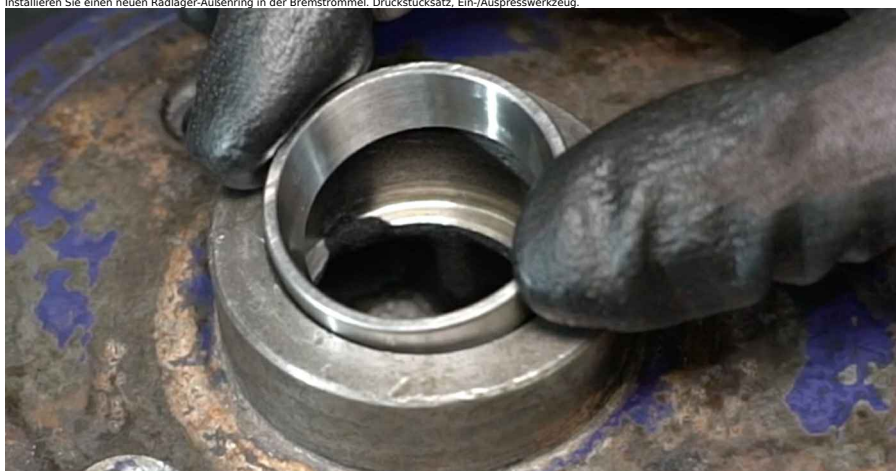
19 Setzen Sie den neuen Innenring des Radlagers in die Bremstrommel ein. Druckstücksatz, Ein-/Auspresswerkzeug.
