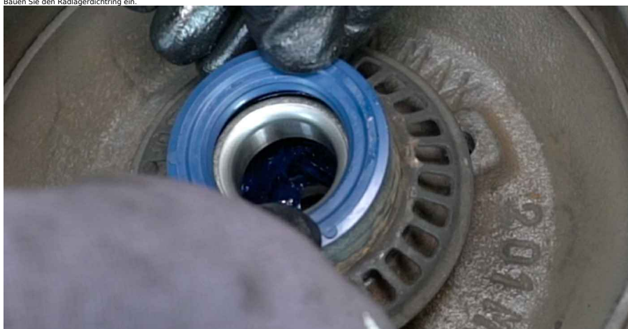
23 Behandeln Sie den Achszapfen. Verwenden Sie Allzweckreinigungsspray. Verwenden Sie Lagerfett.
