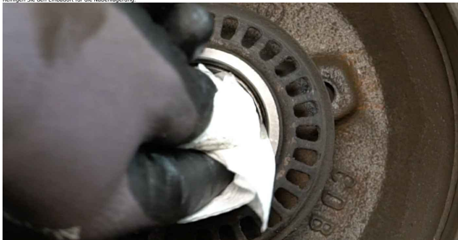
15 Entfernen Sie den Innenring des Radlagers von der Bremstrommel. Verwenden Sie einen Universalabzieher.
